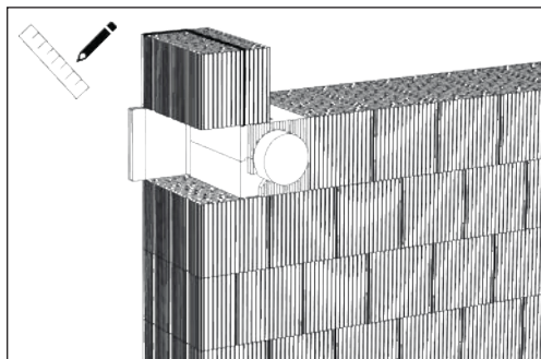
3. Stein für Laibungsabschluss anzeichnen
