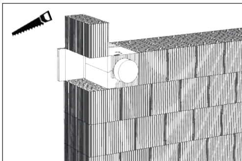
4. Stein für Laibungsabschluss zurechtschneiden
