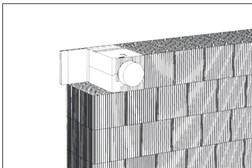
2. Mauerblock und Laibungselement setzen
