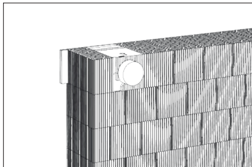
5. Stein für Laibungsabschluss setzen
