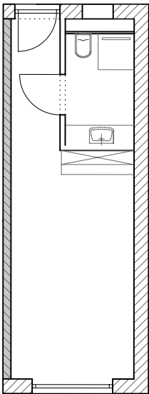
Planungsbeispiel: 1-Zimmer-Wohnung
