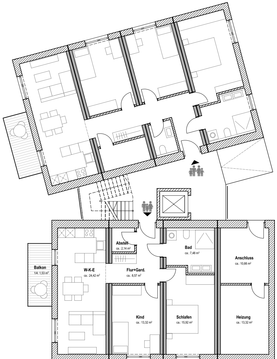
Planungsbeispiel: 4-Zimmer- und 3-Zimmer-Wohnung im Erdgeschoss
